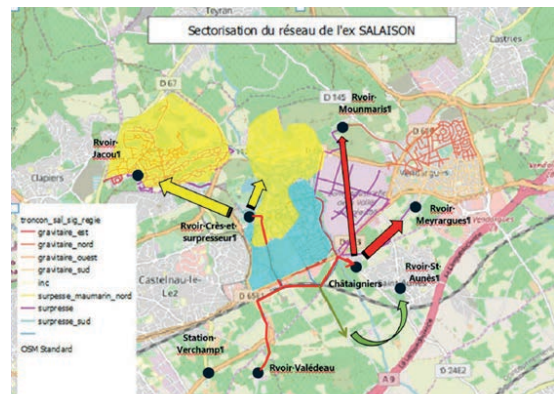
Carte de fonctionnement du réseau du Salaison à partir du réservoir de Valédeau
